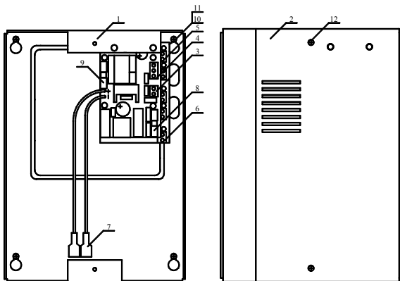
Схема монтажа для исполнения 1
