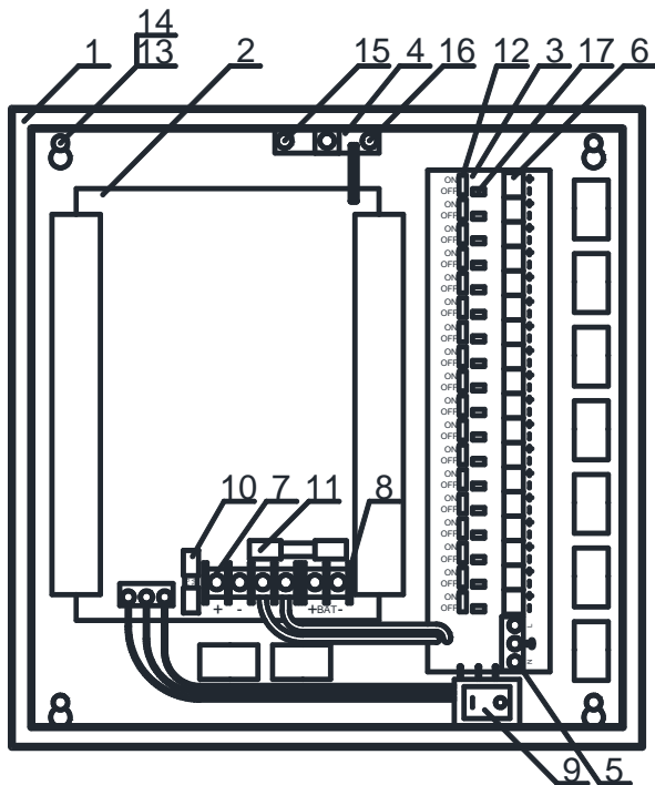
Схема монтажа источника питания ББП-200
